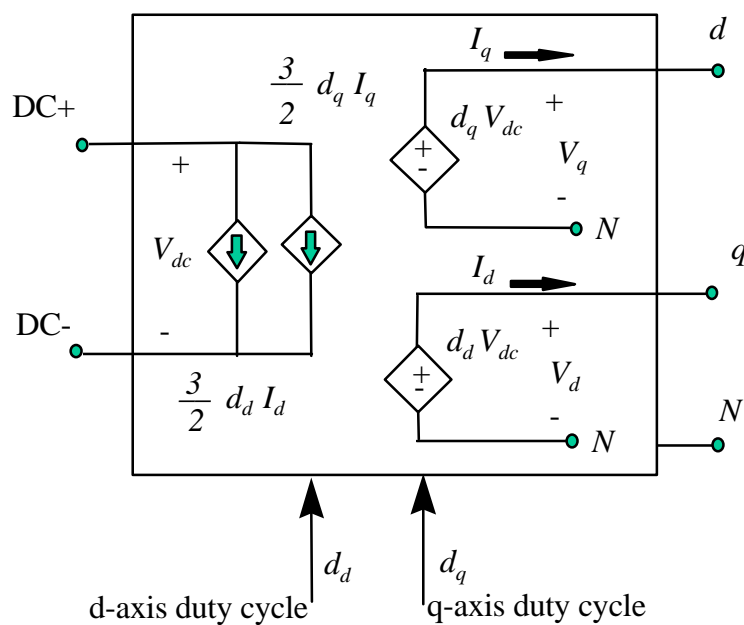
c) DQ average model
