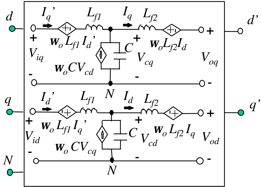
b) DQ model
