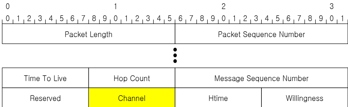
Figure 4.7: OLSR-MC CU message.
